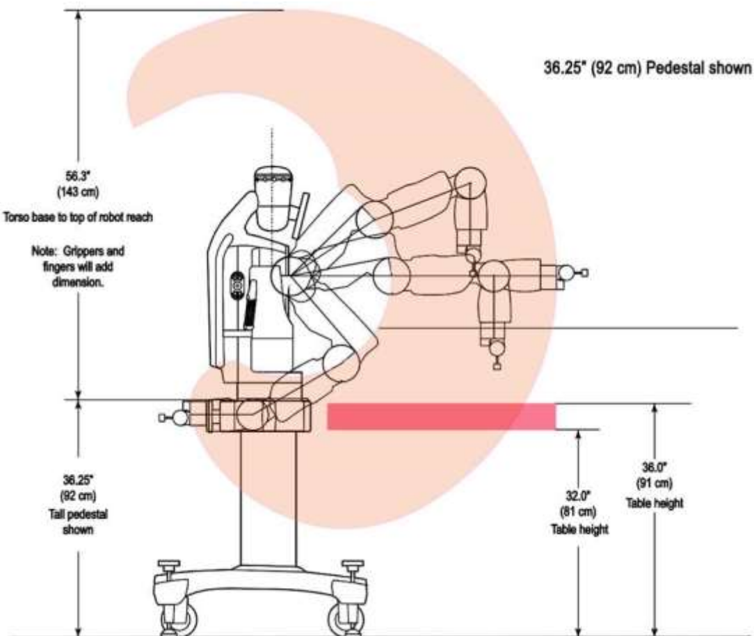
图 1.3 Baxter 侧视图
