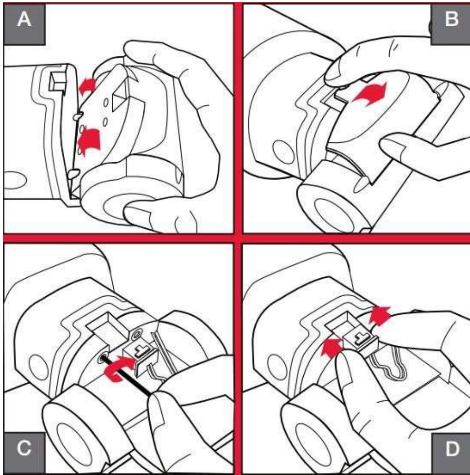
图 1.7 安装电动夹持器底座
