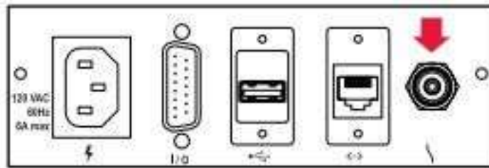
1.13 气泵通过背部气孔（直径 6mm）向机器人提供气源
