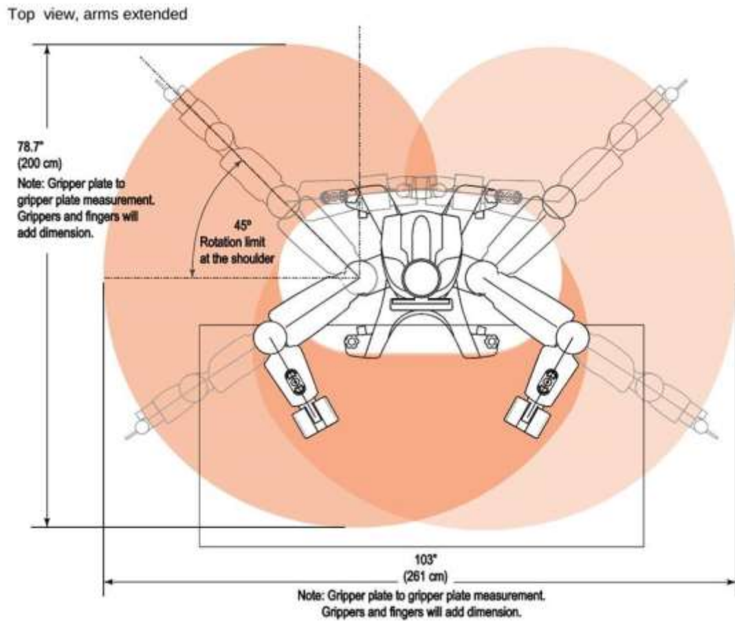
图 1.4 Baxter 机械臂运动范围
