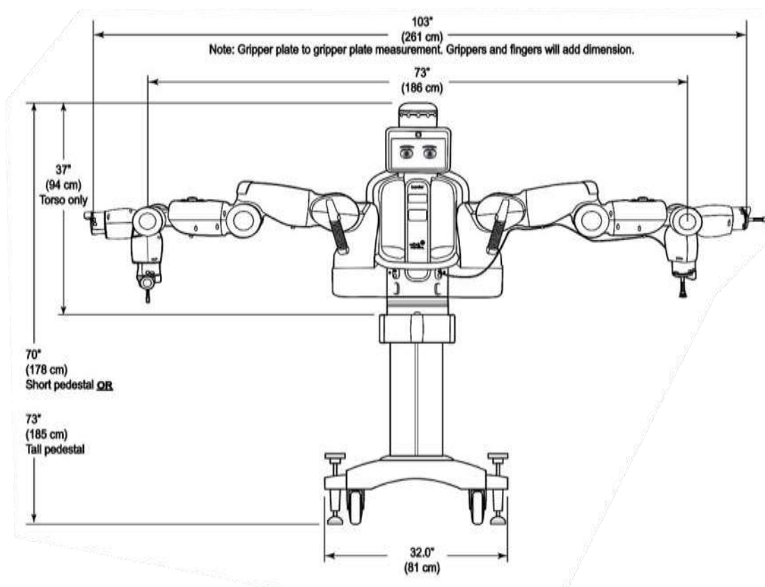
图 1.1 Baxter 正视图
