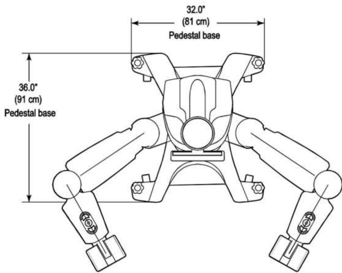
图 1.2 Baxter 俯视图
