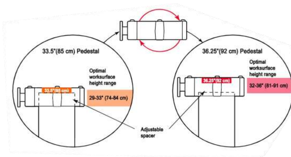
图 1.5 Baxter 底座安装高度
