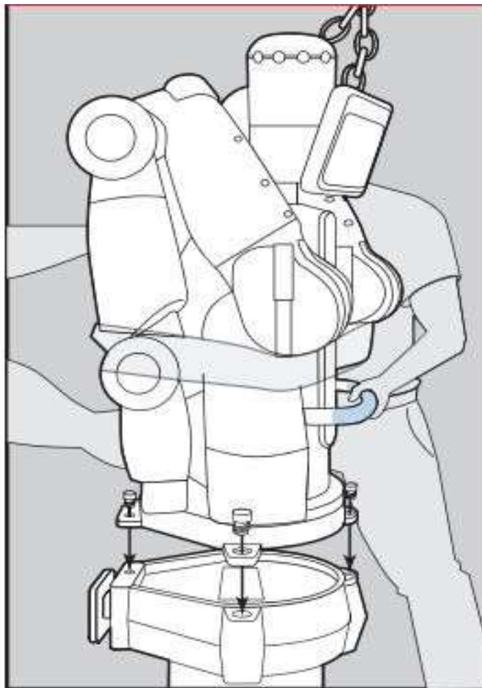
图 1.6 吊装 Baxter
