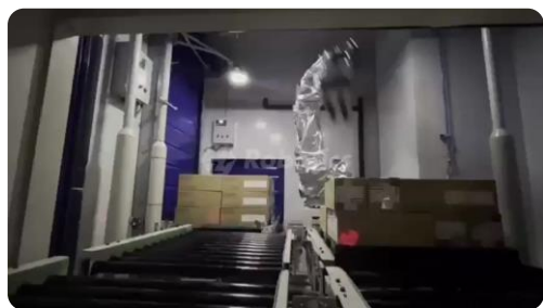
纸箱入库（带扫码）
